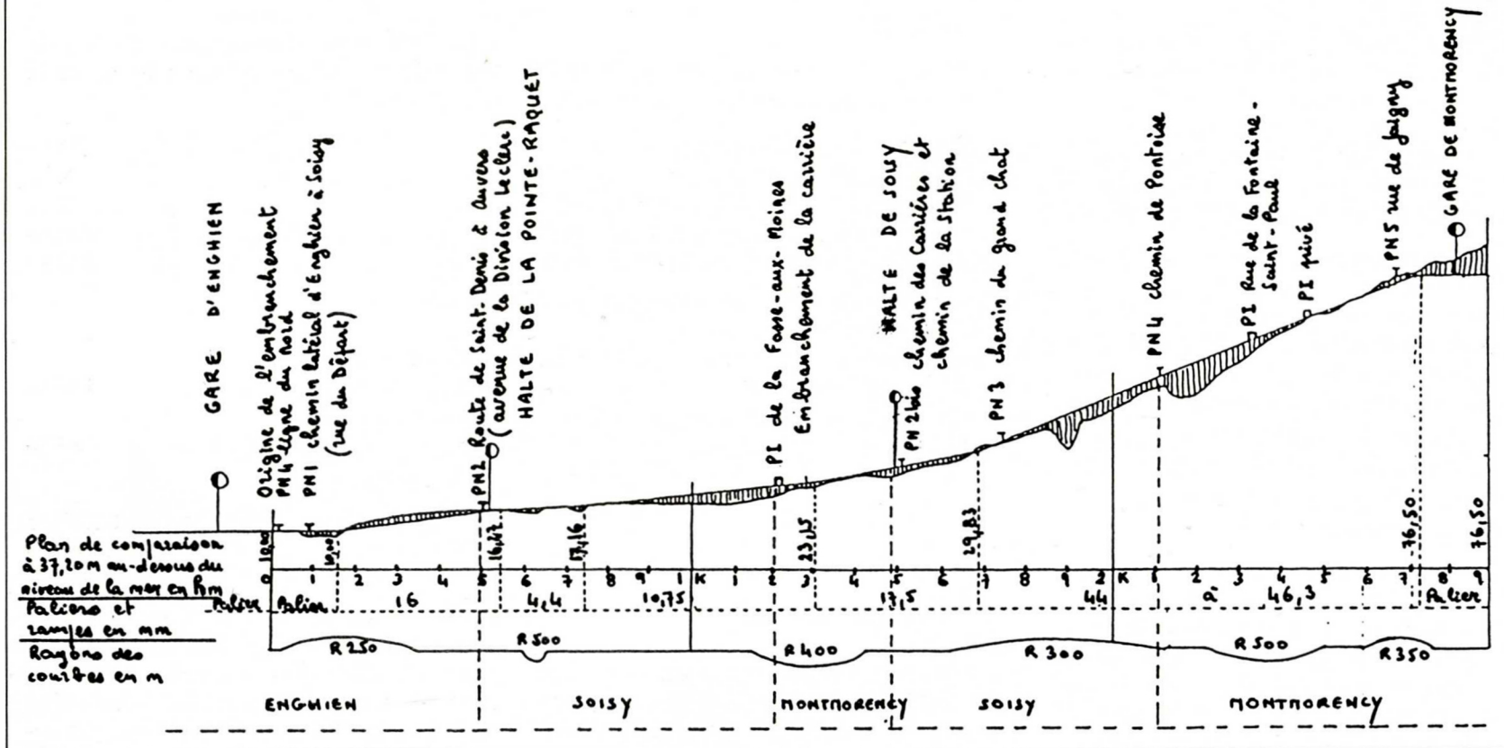
Profil en long de la voie ferrée
